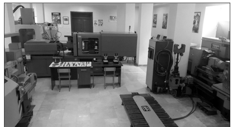
Üç RPI dəzgahından və sənaye robotundan ibarət Robotlaşdırılmış texnoloji kompleks
